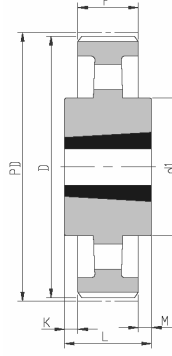
Tip T10
